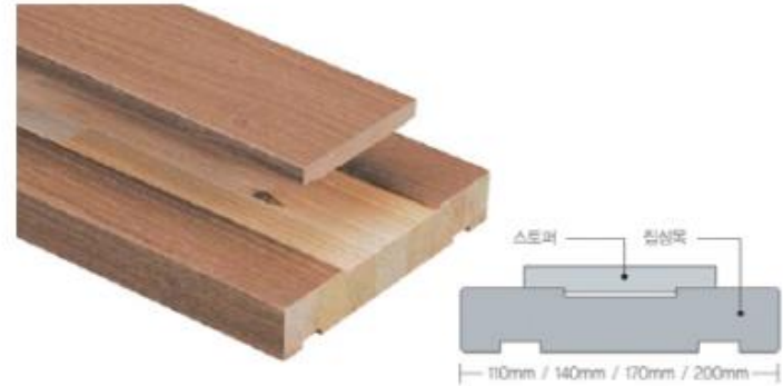
WRAP-integrate
